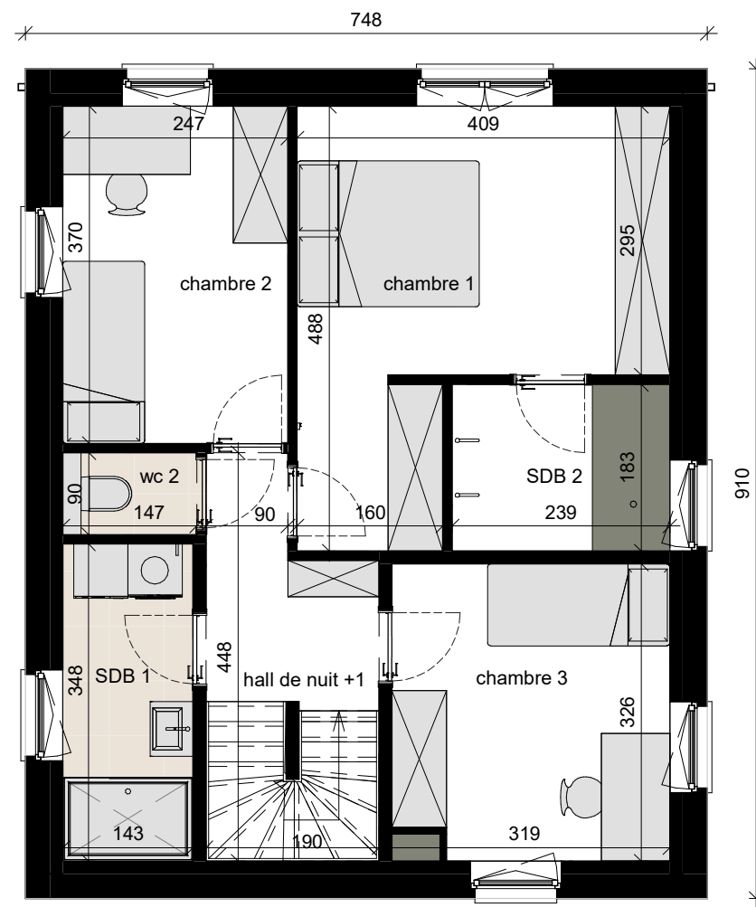
étage surf. brute 68.07 m²
