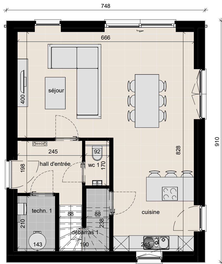
rez-de-chaussée surf. brute 68.07 m²
